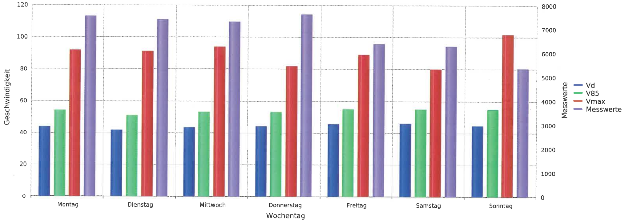
5330 Bad Zurzach, Bruggerstrasse Höhe Baustelle Tunnel, beide Richtungen, 50 km/h Beschränkung Vd, V85, Vmax, Anzahl der Messwerte vs. Wochentag
