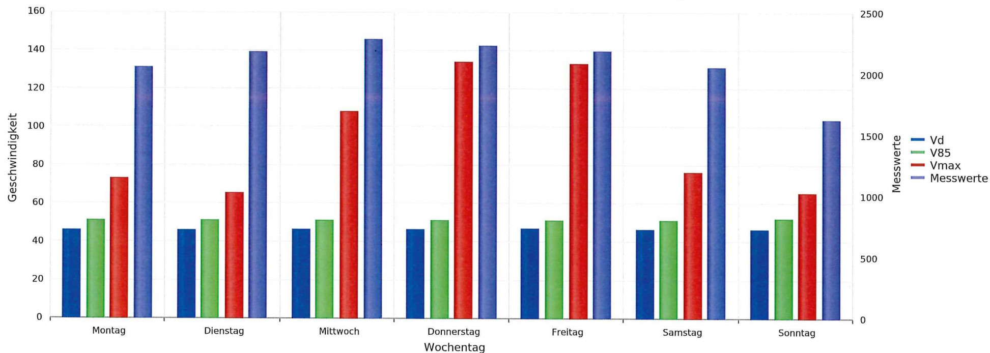
Siglistorf, Hauptstrasse, Fahrtrichtung Mellstorf, 50km/h Beschränkung Vd, V85, Vmax, Anzahl der Messwerte vs. Wochentag
