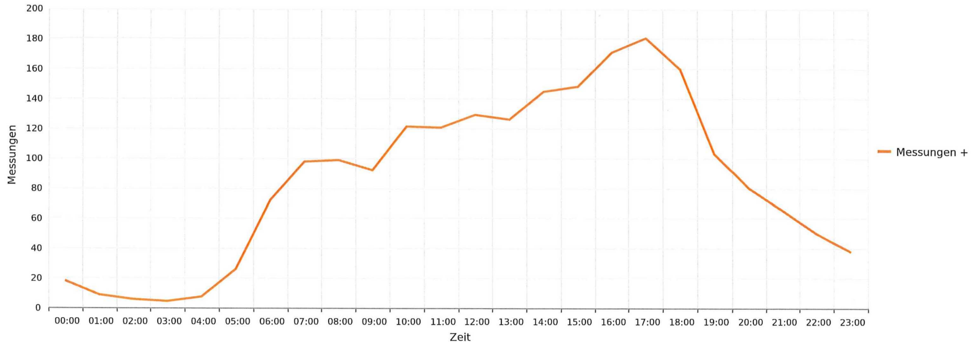
Siglistorf, Hauptstrasse, Fahrtrichtung Mellstorf, 50km/h Beschränkung Gemittelte Anzahl an Messwerten vs. Uhrzeit
