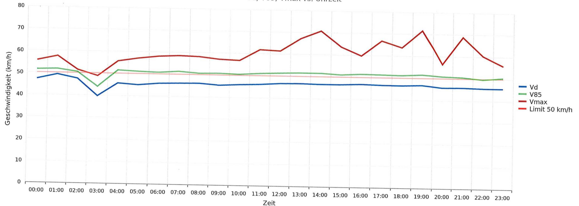
Siglistorf, Hauptstrasse, Fahrtrichtung Mellstorf, 50km/h Beschränkung Vd, V85, Vmax vs. Uhrzeit
