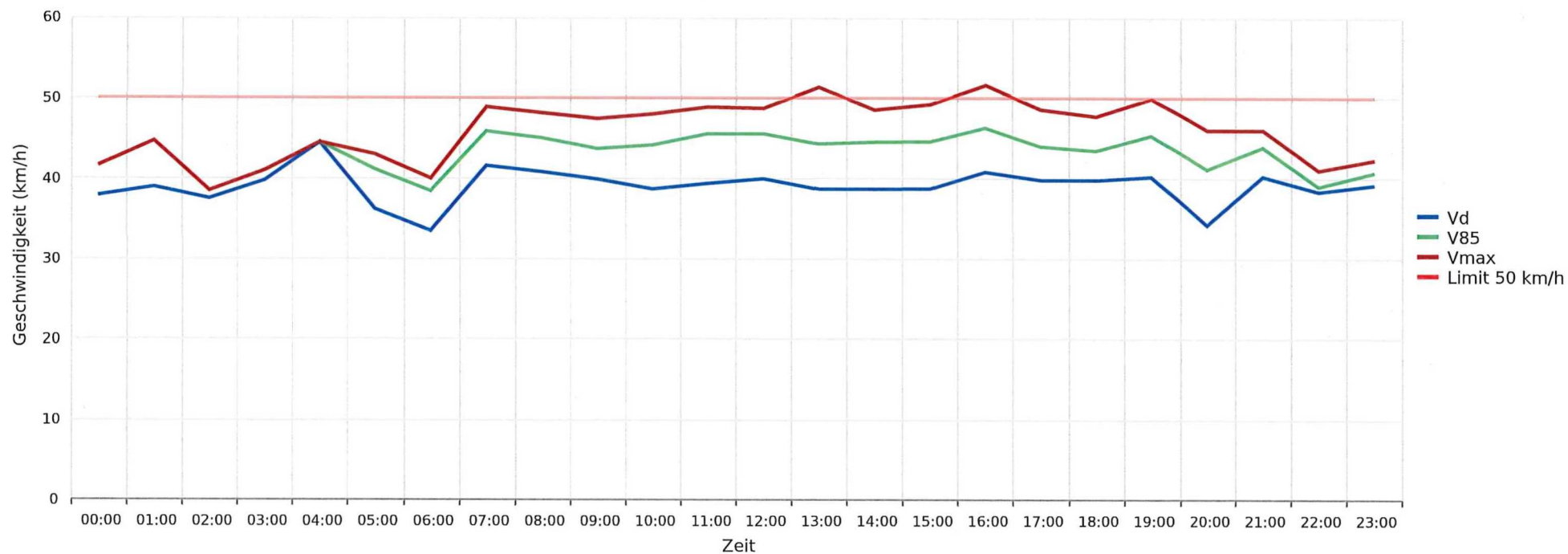
Mandach, Hauptstrasse, Fahrtrichtung Leuggern, 50km/h Beschränkung Vd, V85, Vmax vs. Uhrzeit
