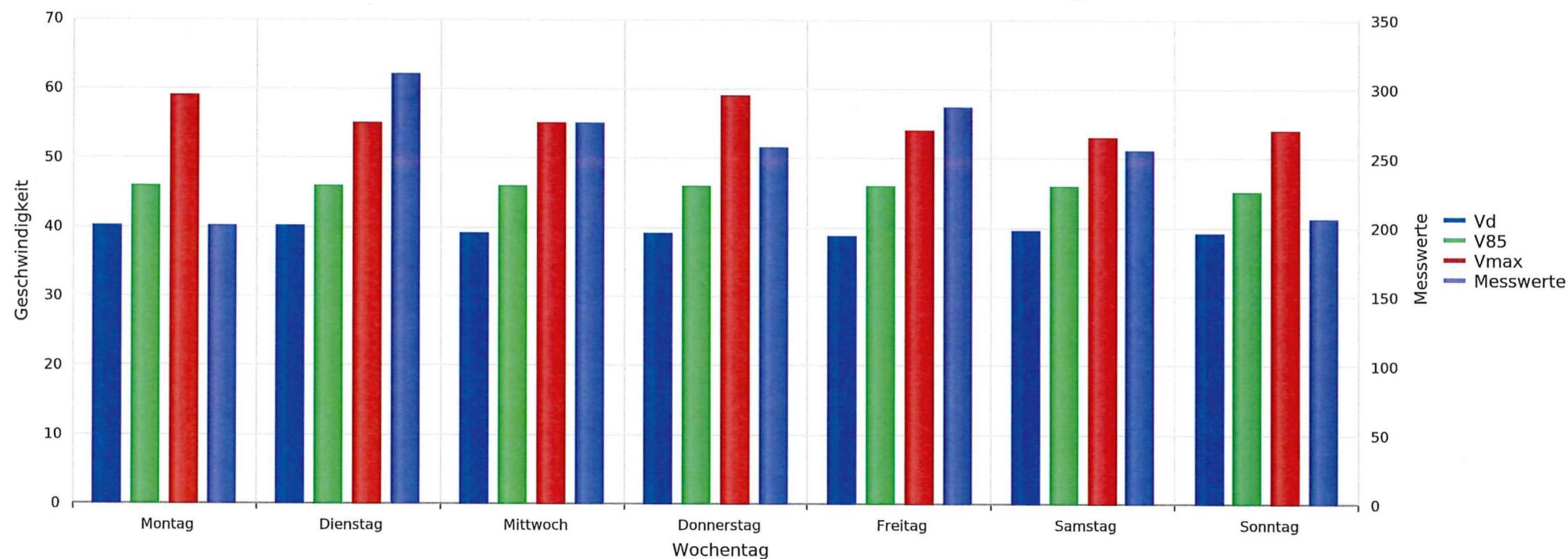
Mandach, Hauptstrasse, Fahrtrichtung Leuggern, 50km/h Beschränkung Vd, V85, Vmax, Anzahl der Messwerte vs. Wochentag
