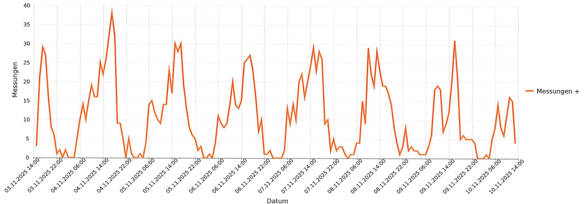
Mandach, Hauptstrasse, Fahrtrichtung Leuggern, 50km/h Beschränkung Anzahl der Messwerte vs. Messzeitraum
