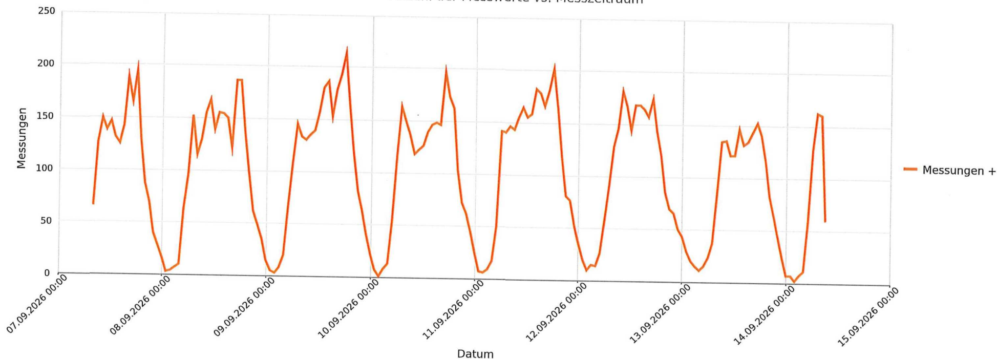
Döttingen, Surbtalstrasse, Fahrtrichtung Döttingen, 50km/h Beschränkung Anzahl der Messwerte vs. Messzeitraum
