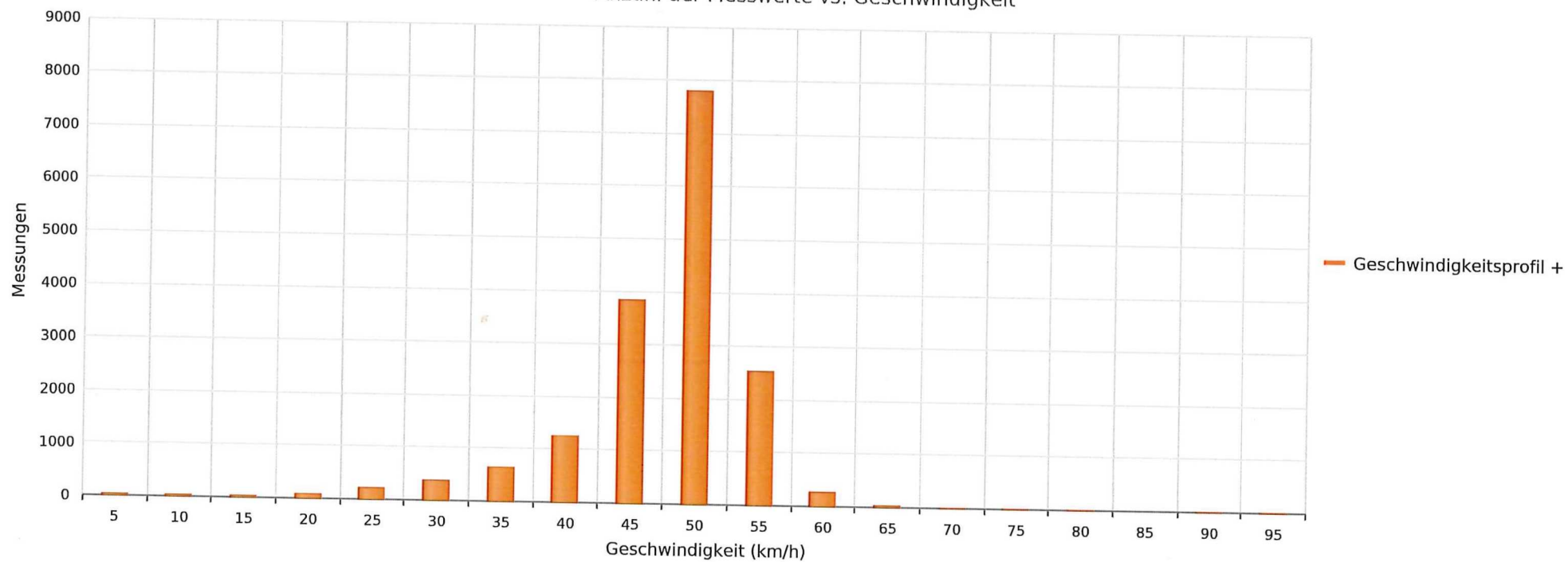
Döttingen, Surbtalstrasse, Fahrtrichtung Döttingen, 50km/h Beschränkung Anzahl der Messwerte vs. Geschwindigkeit
