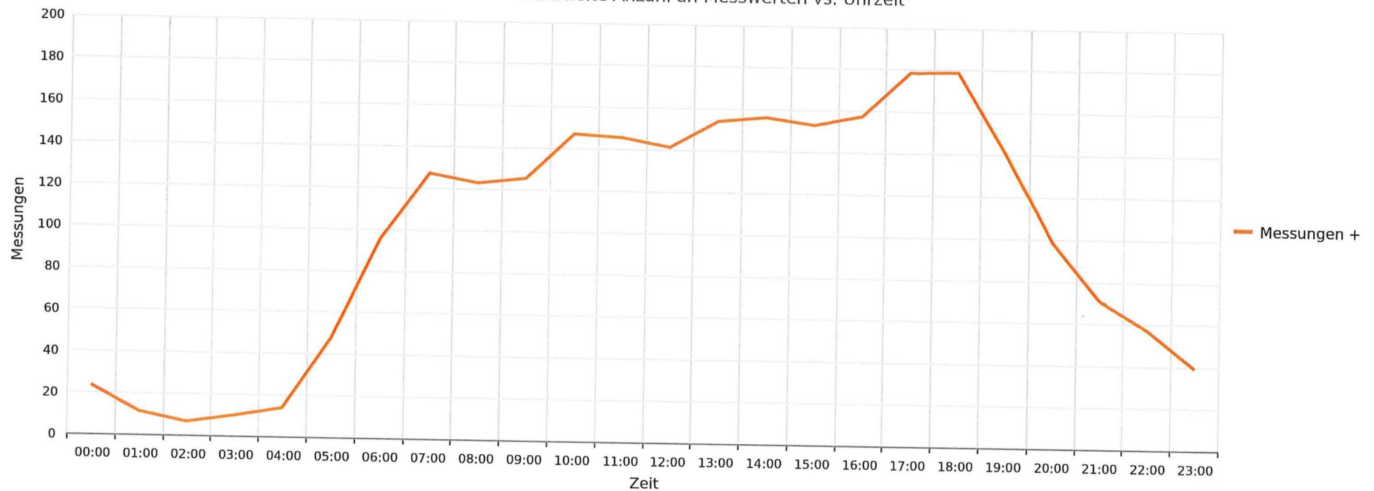
Döttingen, Surbtalstrasse, Fahrtrichtung Döttingen, 50km/h Beschränkung Gemittelte Anzahl an Messwerten vs. Uhrzeit
