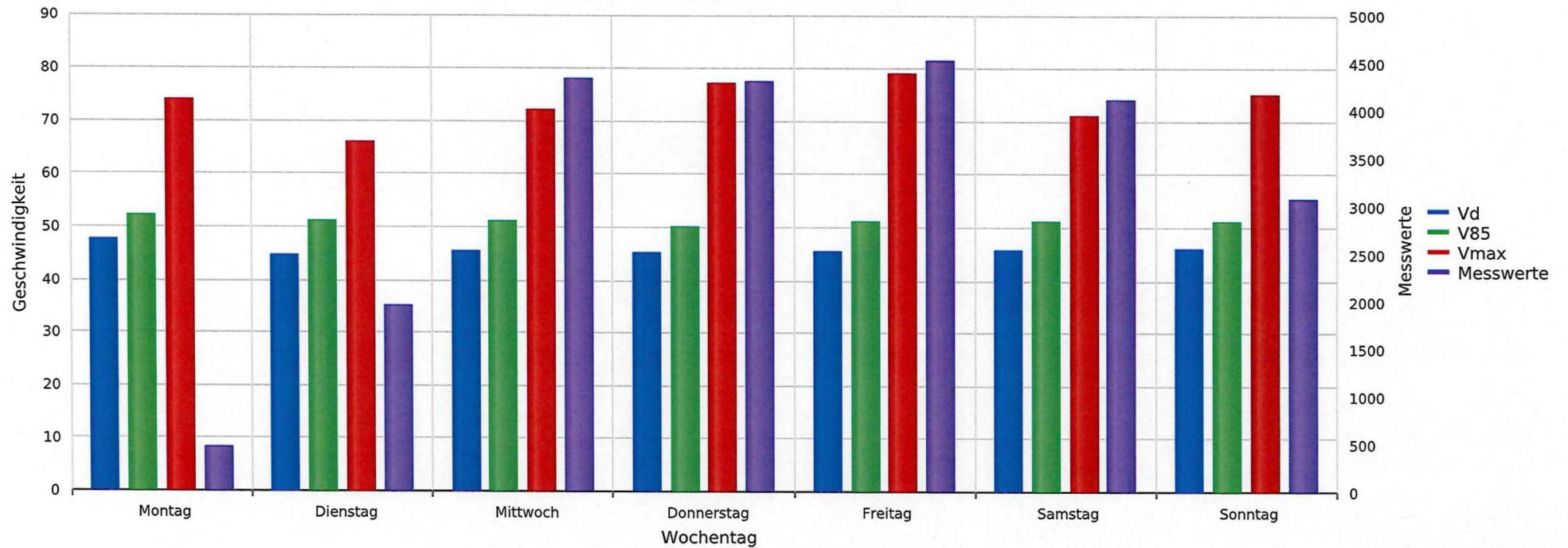
Kleindöttingen, Hauptstrasse, Fahrtrichtung Böttstein, 50 km/h Beschränkung Vd, V85, Vmax, Anzahl der Messwerte vs. Wochentag
