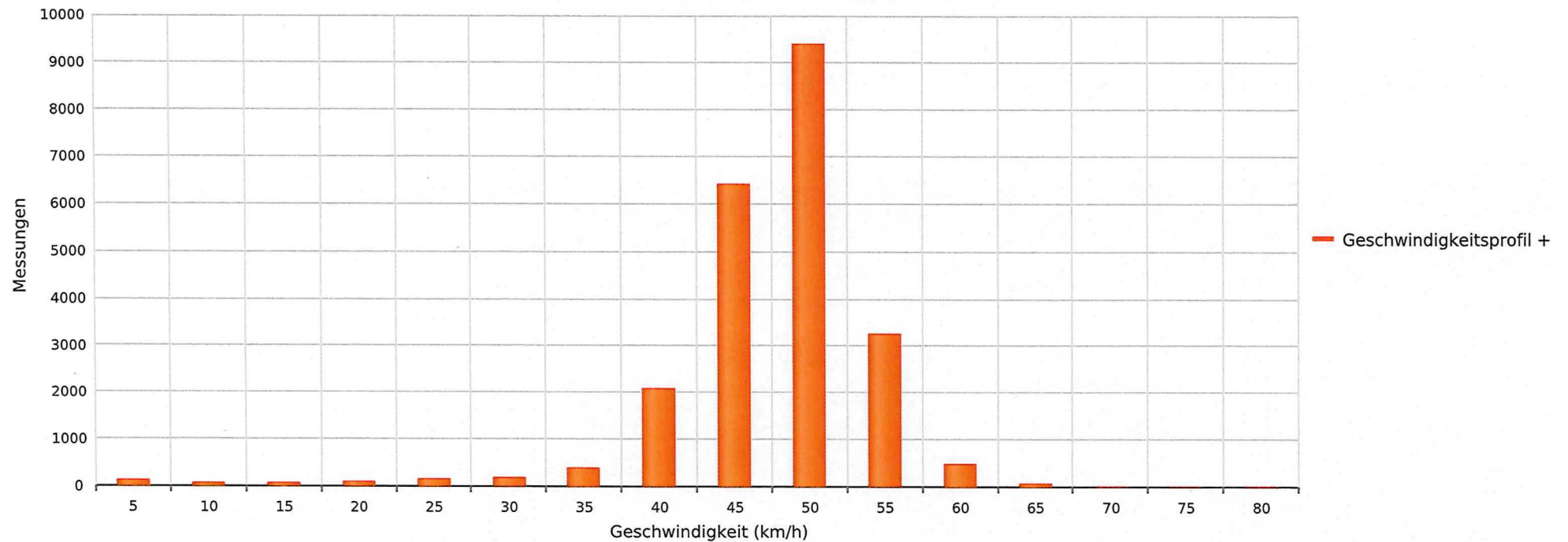
Kleindöttingen, Hauptstrasse, Fahrtrichtung Böttstein, 50 km/h Beschränkung Anzahl der Messwerte vs. Geschwindigkeit
