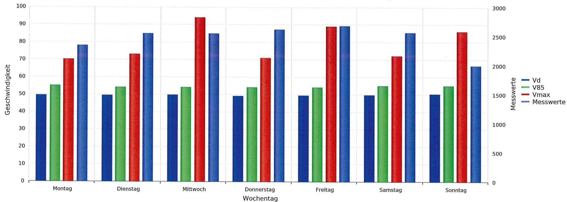
Endingen, Surbtalstrasse, Fahrtrichtung Tegerfelden, 50km/h Beschränkung Vd, V85, Vmax, Anzahl der Messwerte vs. Wochentag
