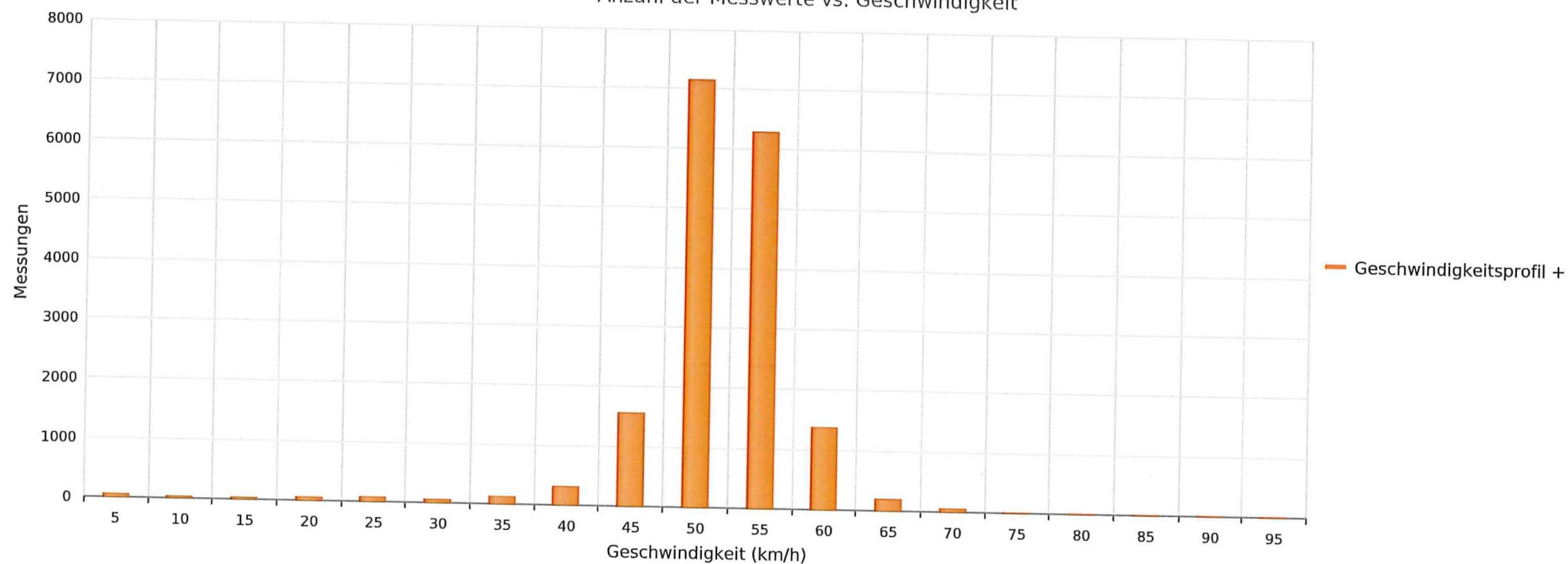
Endingen, Surbtalstrasse, Fahrtrichtung Tegerfelden, 50km/h Beschränkung Anzahl der Messwerte vs. Geschwindigkeit
