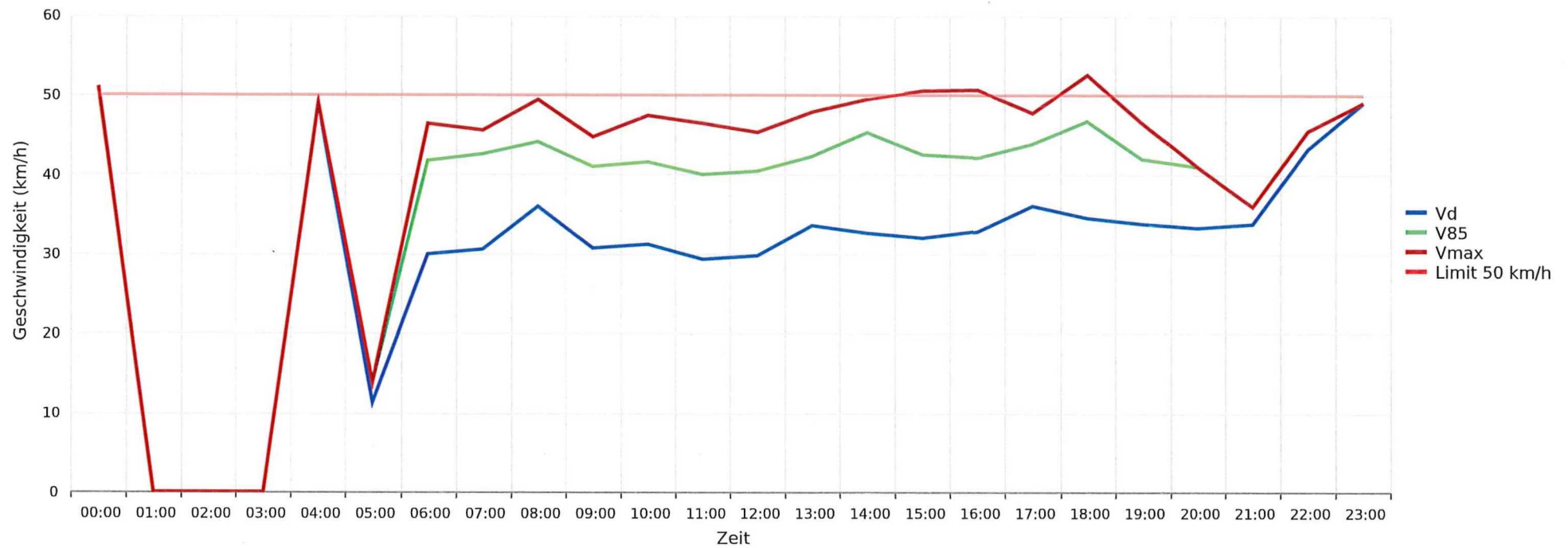
Leuggern, Schlatterstrasse, Fahrtrichtung Tal, 50km/h Beschränkung Vd, V85, Vmax vs. Uhrzeit
