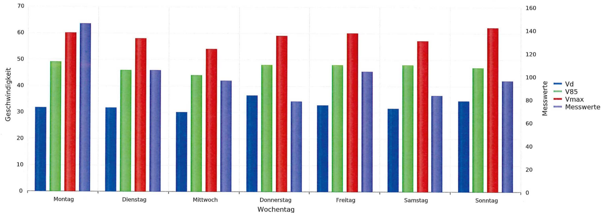
Leuggern, Schlatterstrasse , Fahrtrichtung Tal, 50km/h Beschränkung Vd, V85, Vmax, Anzahl der Messwerte vs. Wochentag
