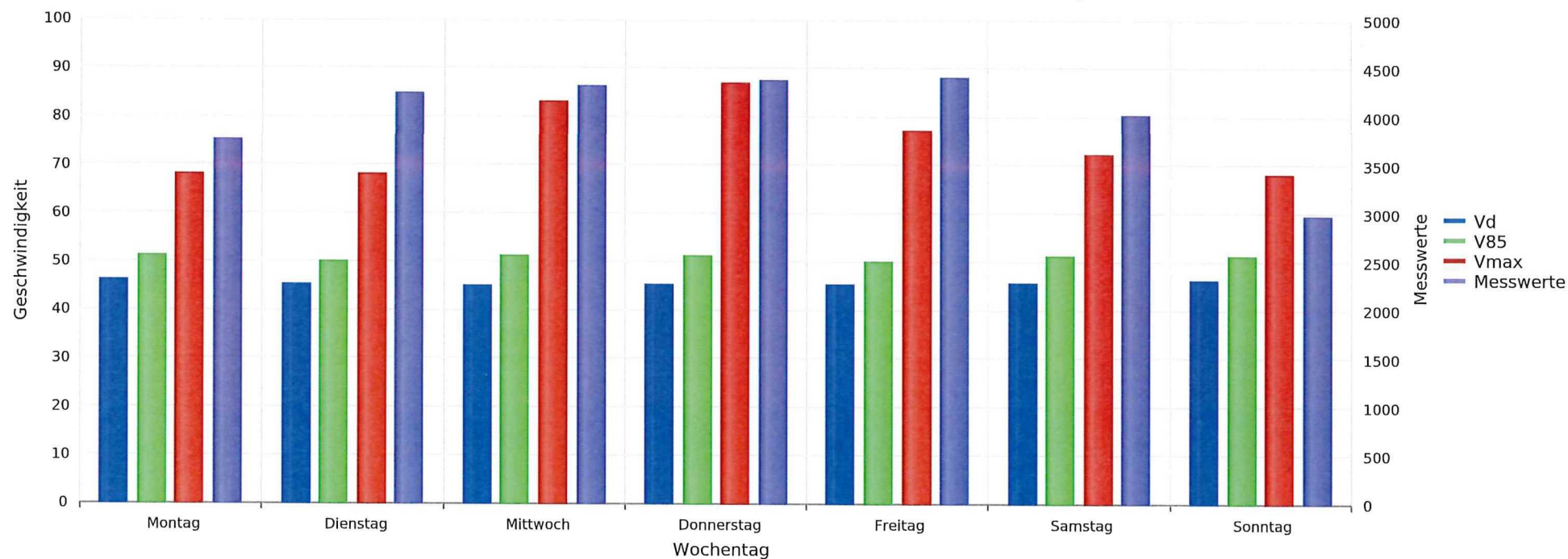
Kleindöttingen, Hauptstrasse, Fahrtrichtung Leuggern, 50km/h Beschränkung Vd, V85, Vmax, Anzahl der Messwerte vs. Wochentag
