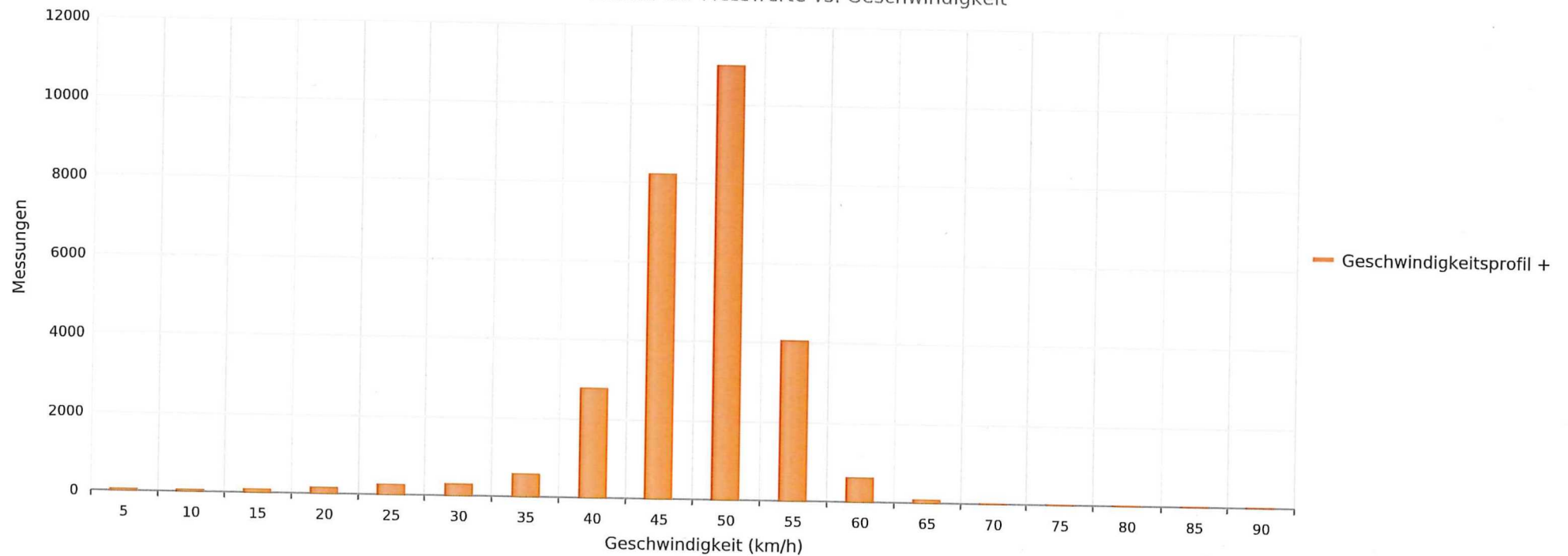
Kleindöttingen, Hauptstrasse, Fahrtrichtung Leuggern, 50km/h Beschränkung Anzahl der Messwerte vs. Geschwindigkeit
