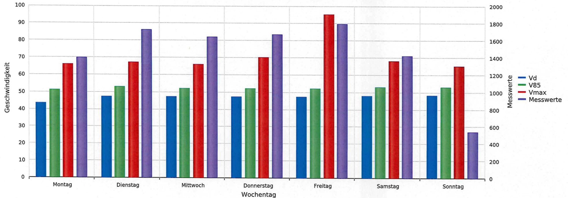
Endingen, Hirschengasse, Fahrtrichtung Endingen, 50km/h Beschränkung Vd, V85, Vmax, Anzahl der Messwerte vs. Wochentag
