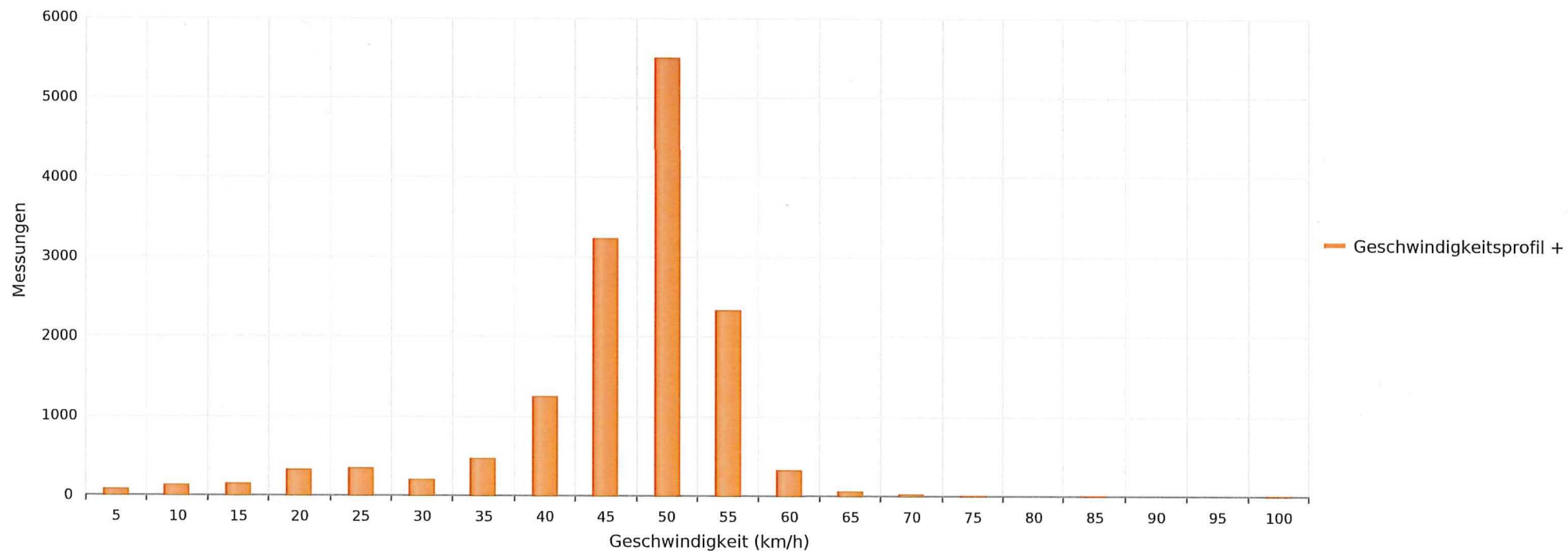
Kleindöttingen, Hauptstrasse, Fahrtrichtung Döttingen, 50km/h Beschränkung Anzahl der Messwerte vs. Geschwindigkeit
