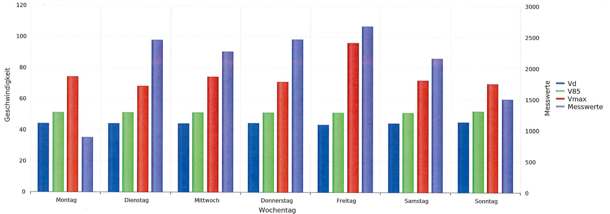
Kleindöttingen, Hauptstrasse, Fahrtrichtung Döttingen, 50km/h Beschränkung Vd, V85, Vmax, Anzahl der Messwerte vs. Wochentag
