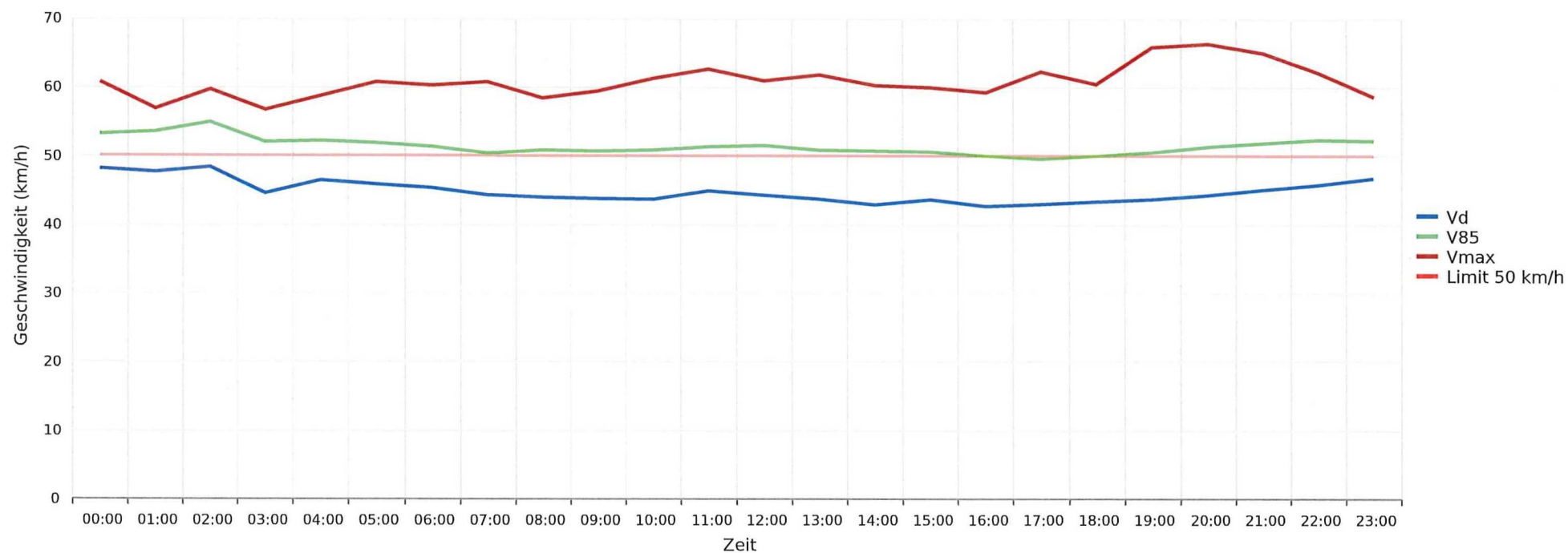
Kleindöttingen, Hauptstrasse, Fahrtrichtung Döttingen, 50km/h Beschränkung Vd, V85, Vmax vs. Uhrzeit
