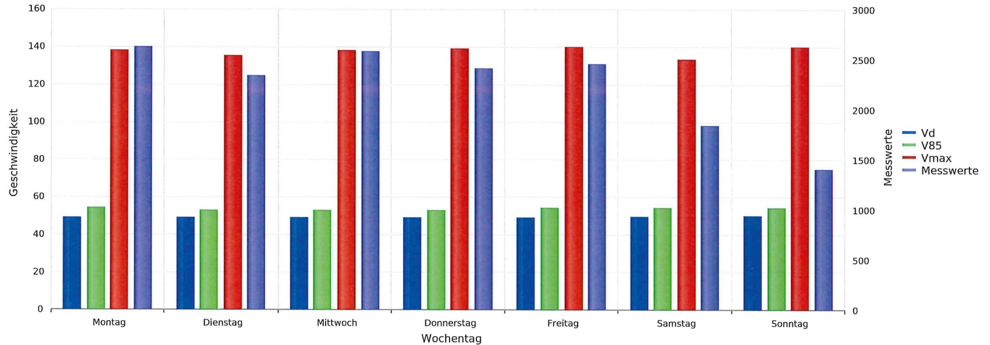
Schneisingen, Landstrasse, Rtg Siglistorf, 50km/h Beschränkung Vd, V85, Vmax, Anzahl der Messwerte vs. Wochentag
